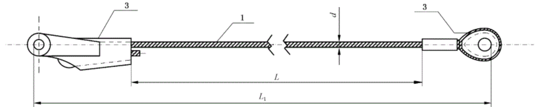
图 A.7 楔形套索具试样
