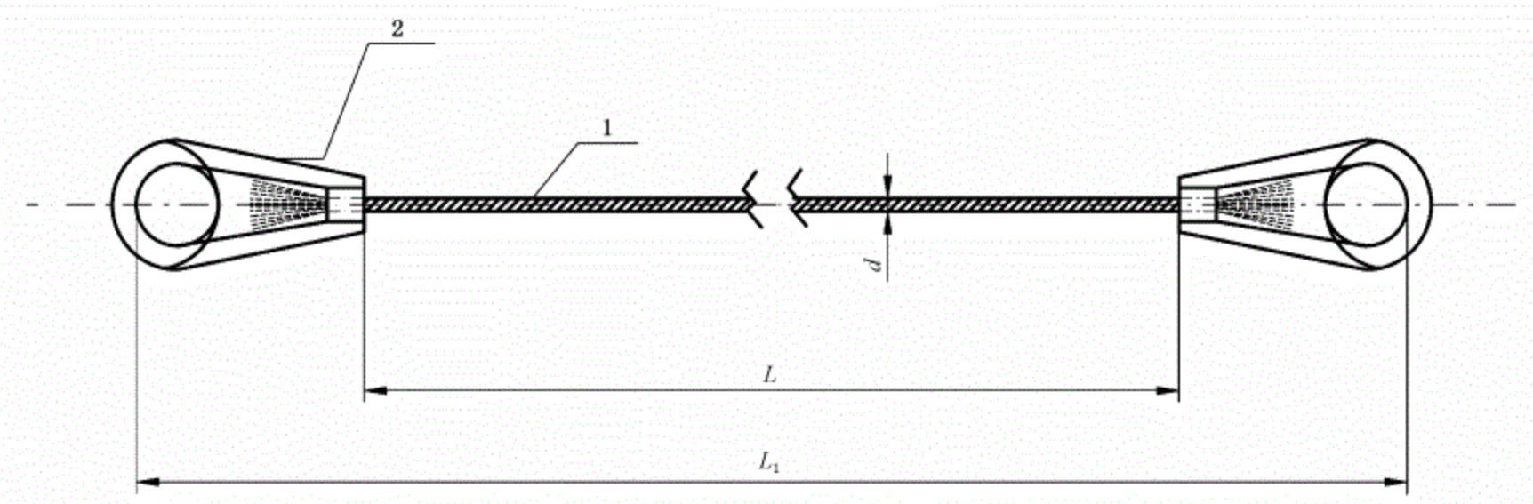
图 A.1 压制固结索具试样
