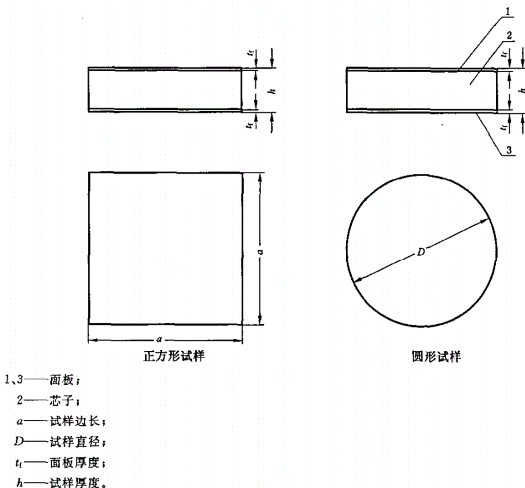
图 2 平压试样
