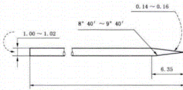
图 1 沥青针入度试验用针
