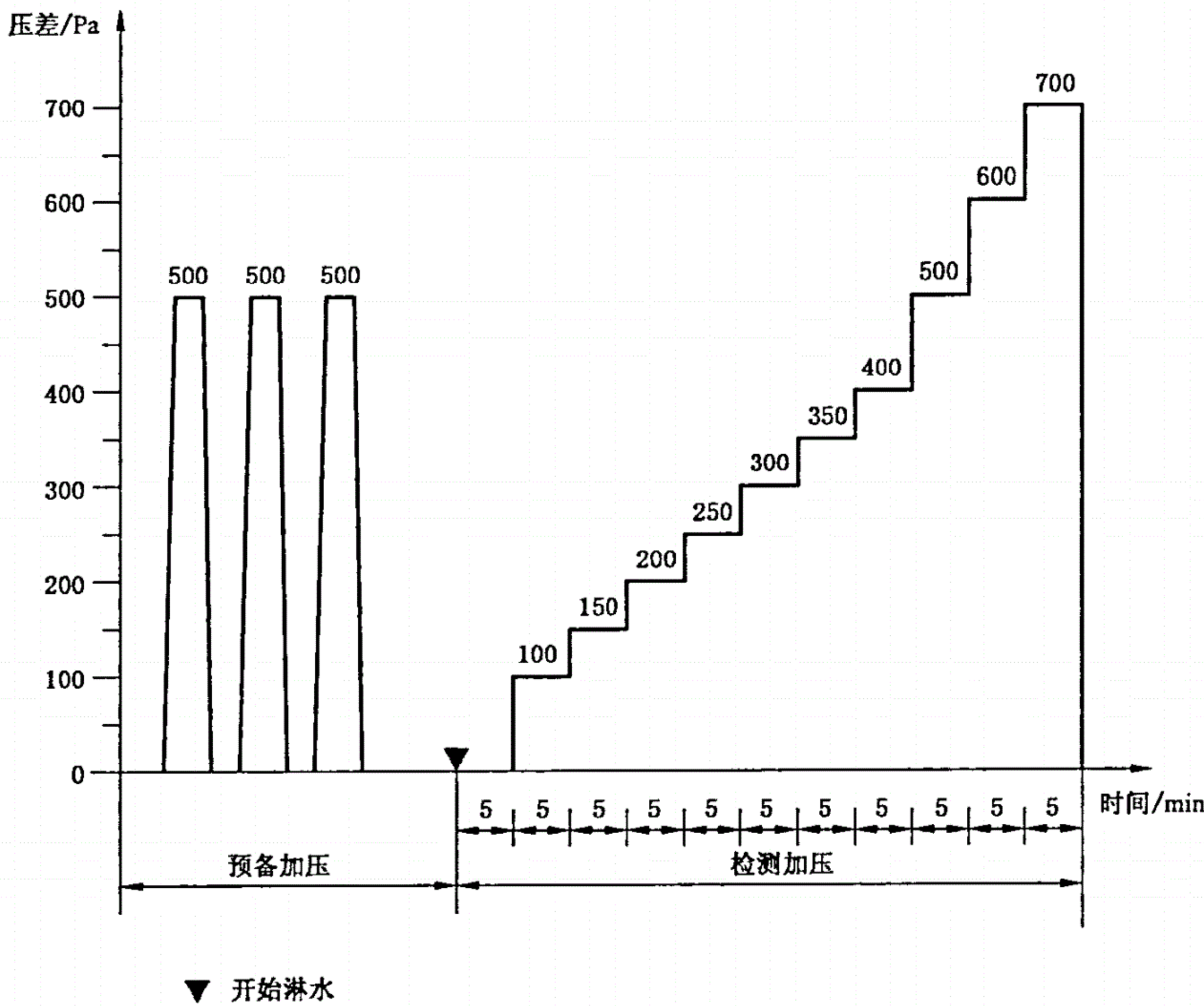
图 4 稳定逐级加压法顺序示意图
